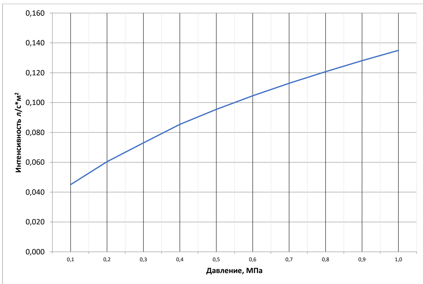
График зависимости интенсивности орошения водой от давления для высоты 2,5 м и площади 3х4 м 2
